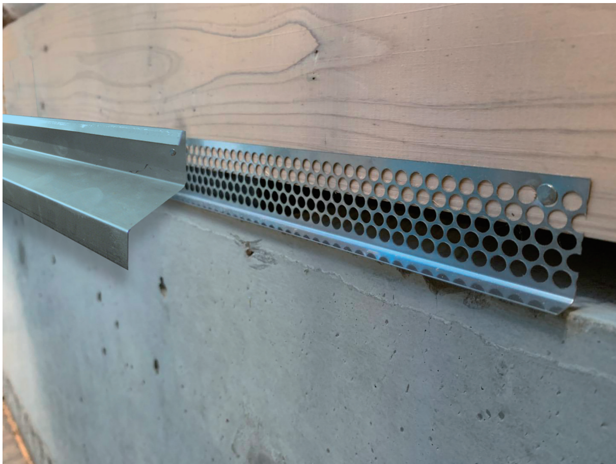
防鼠材施工例（徳島県三好郡）
