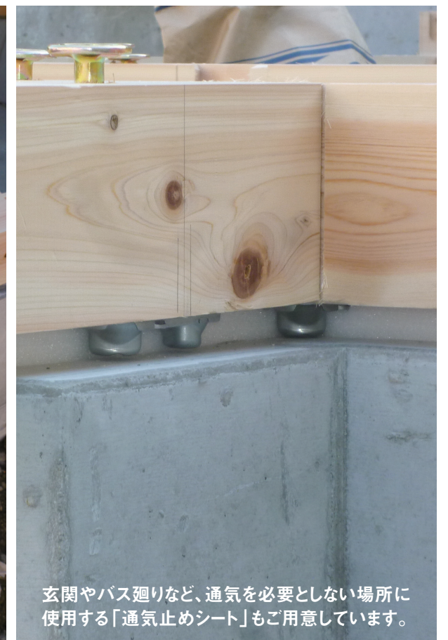
ダイカラットと通気止めシートを使った施工例 (大阪府池田市)
