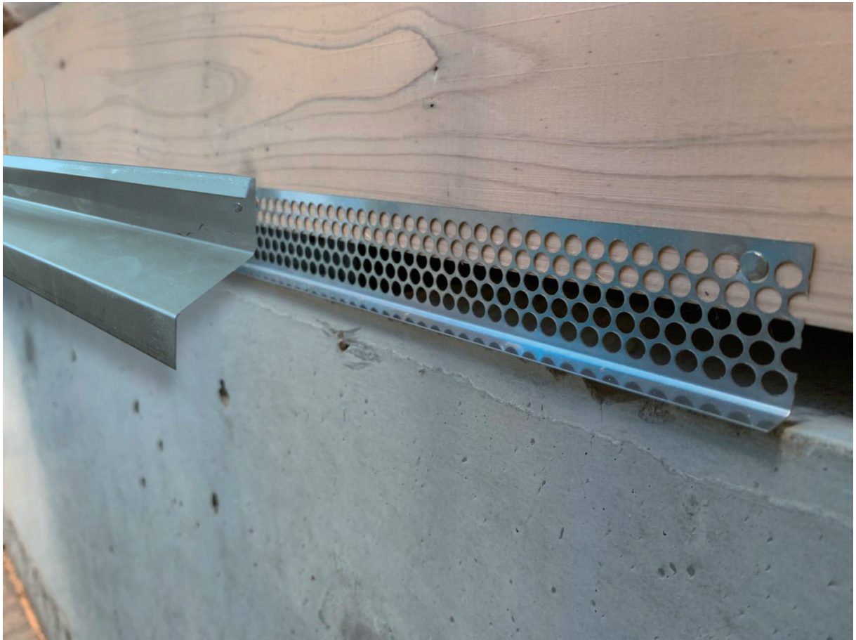
防鼠材・水切り材 施工例（徳島県三好郡）
