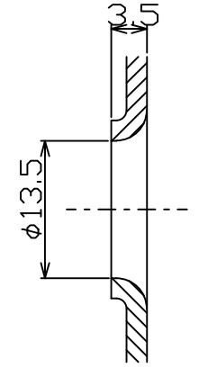
ベアリング部詳細
